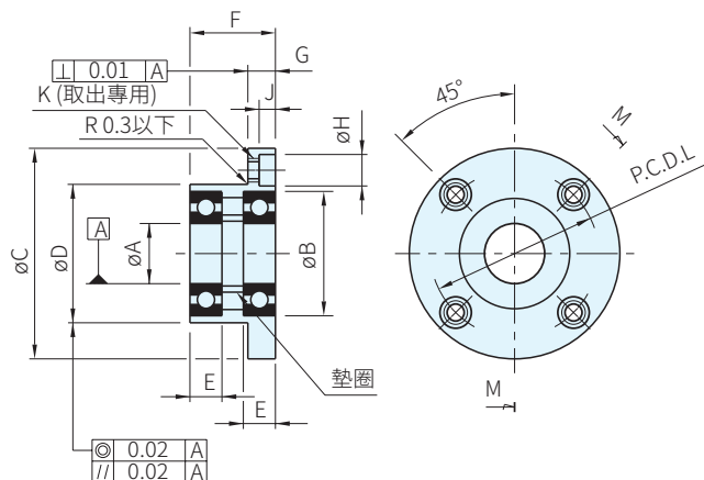
斷面 M-M
